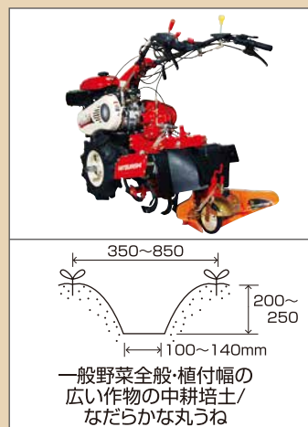
オレンジ培土器 尾輪付
