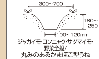
ピンク培土器 尾輪付
