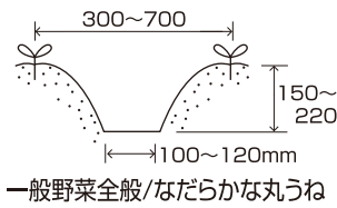
ニューイエロー培土器 尾輪付
