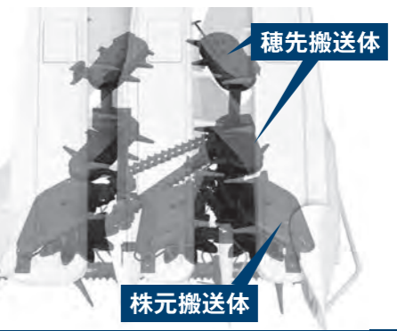
三段かき込み搬送
