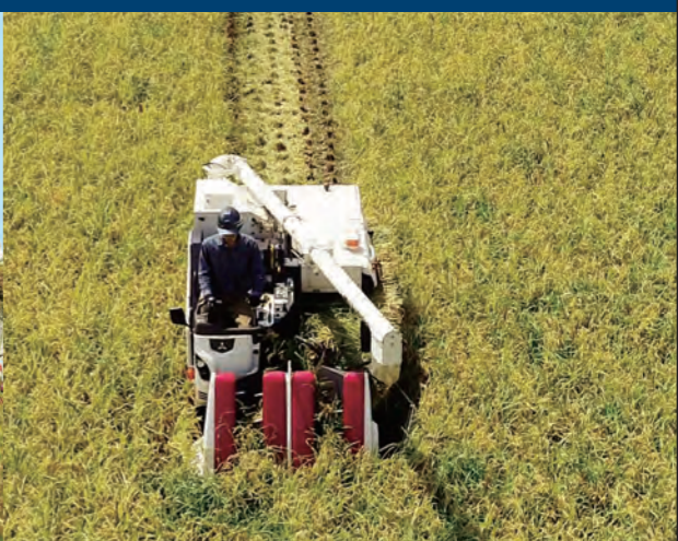
完全全面刈り(V435A)
